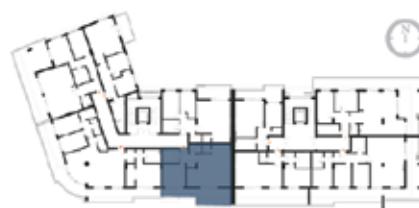
STAN BR. 30 - POVUČENA ETAŽA P=75,35
