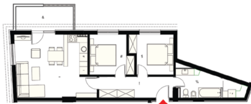
STAN BR. 33 - POVUČENA ETAŽA P=65,28
